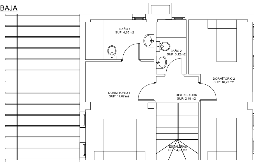
PLANTA PRIMERA
