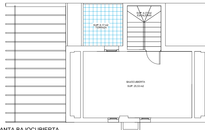
PLANTA BAJOCUBIERTA
