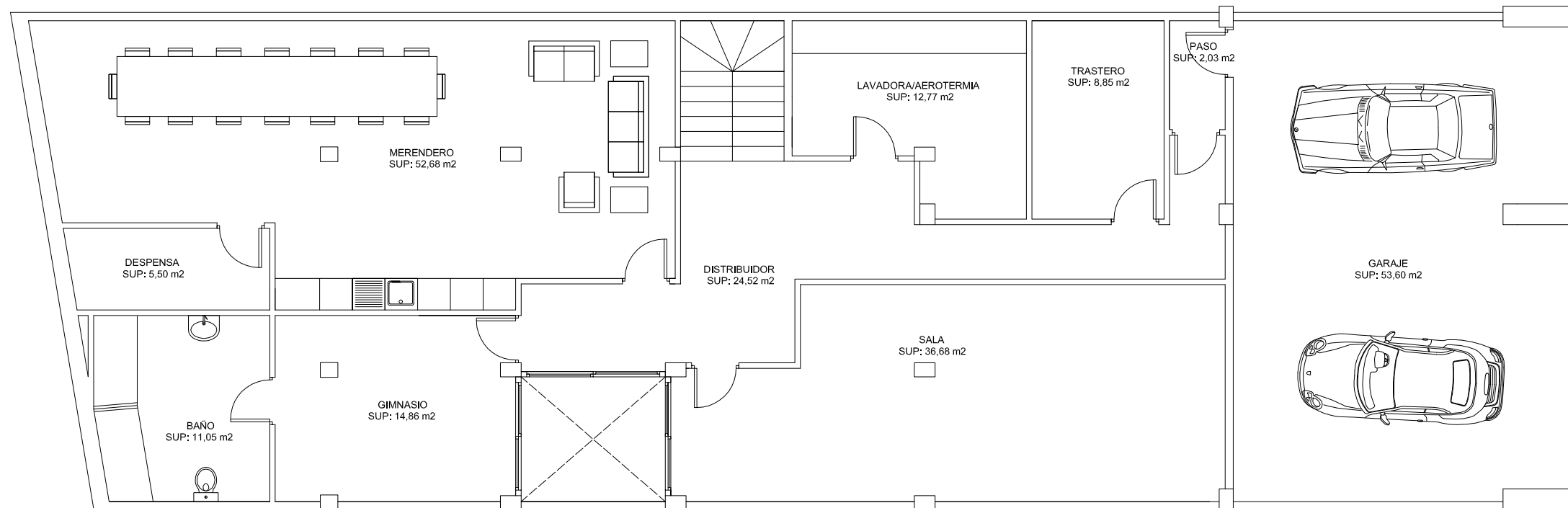
PLANTA SOTANO
