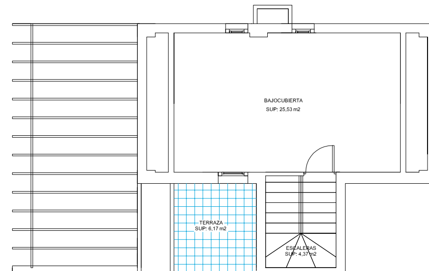
PLANTA BAJOCUBIERTA
