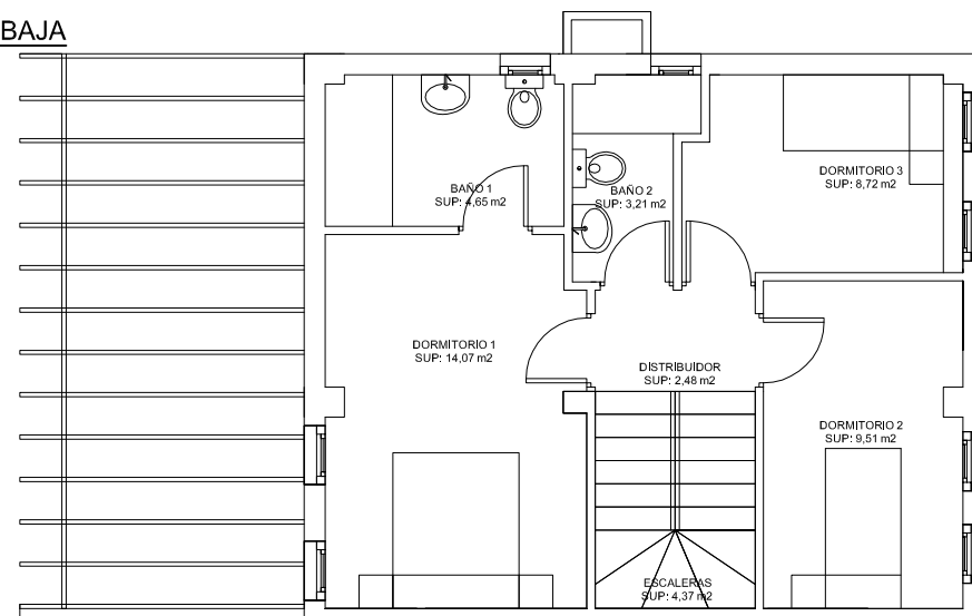
PLANTA PRIMERA
