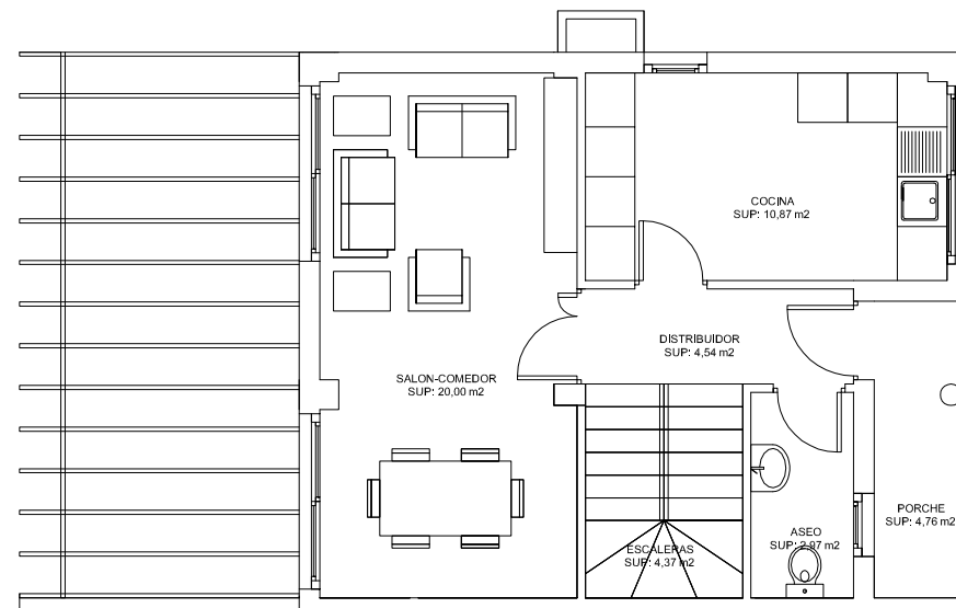
PLANTA BAJA
