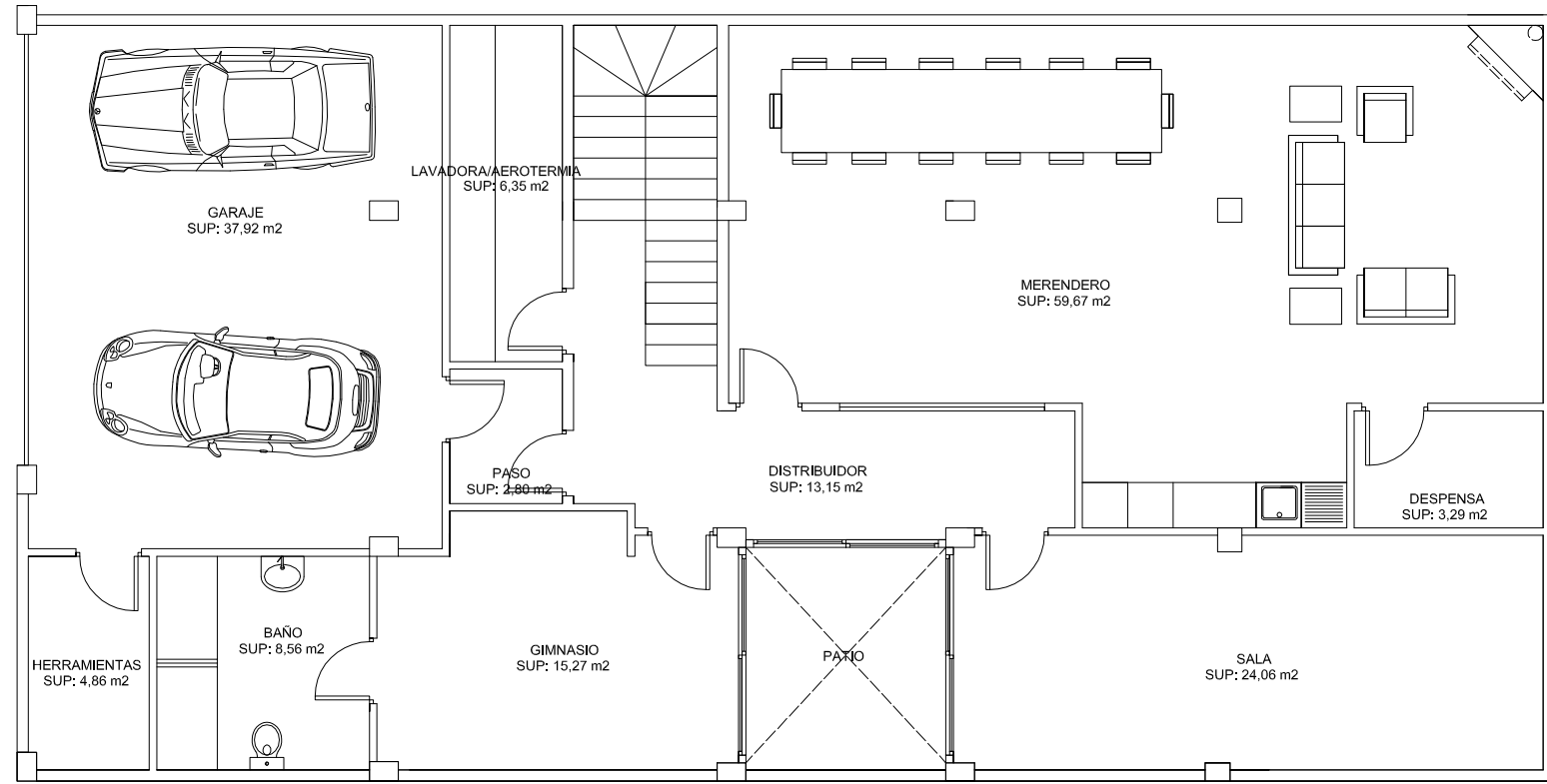
PLANTA SOTANO
