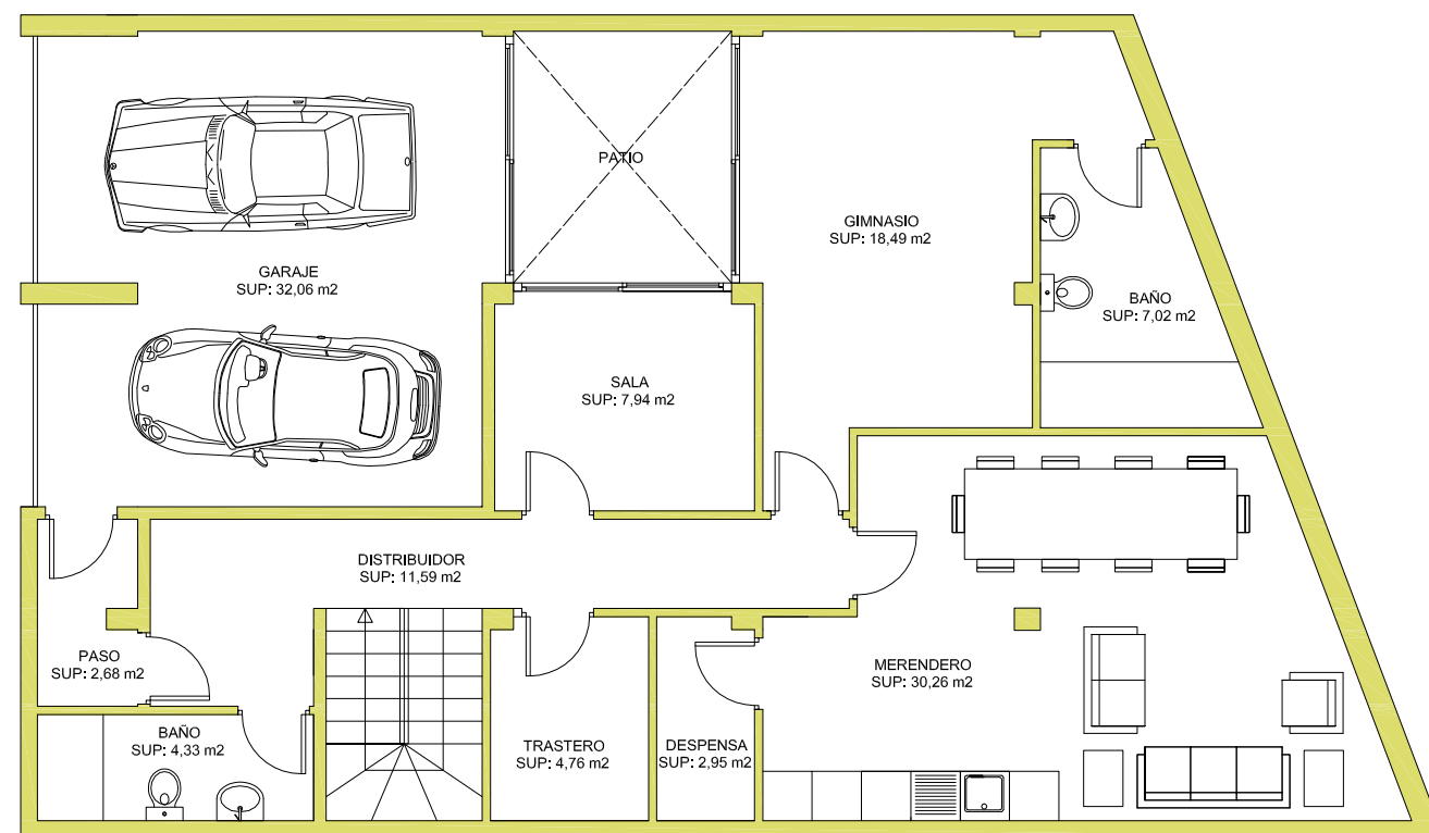
PLANTA SOTANO ESCALA 1:100
